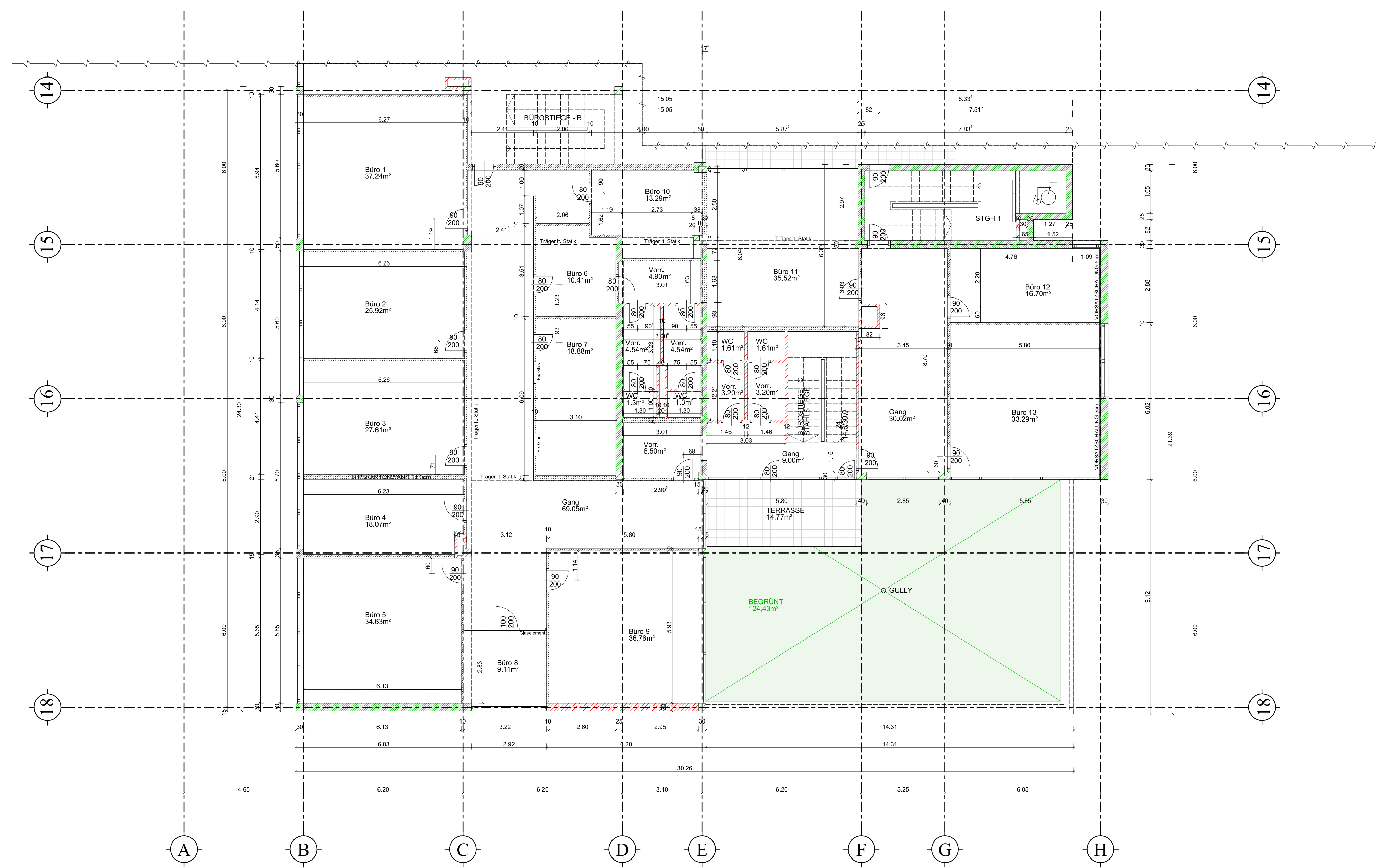
GRUNDRISS 1: OBERGESCHOSS
