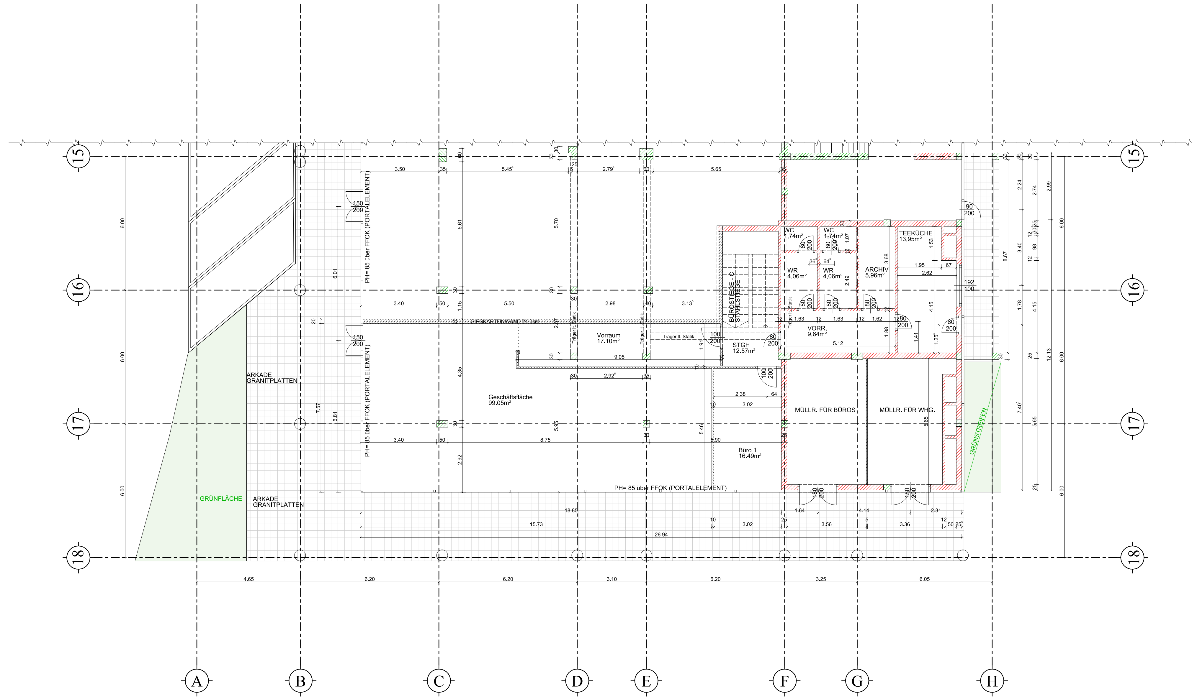
GRUNDRISS ERDGESCHOSS
